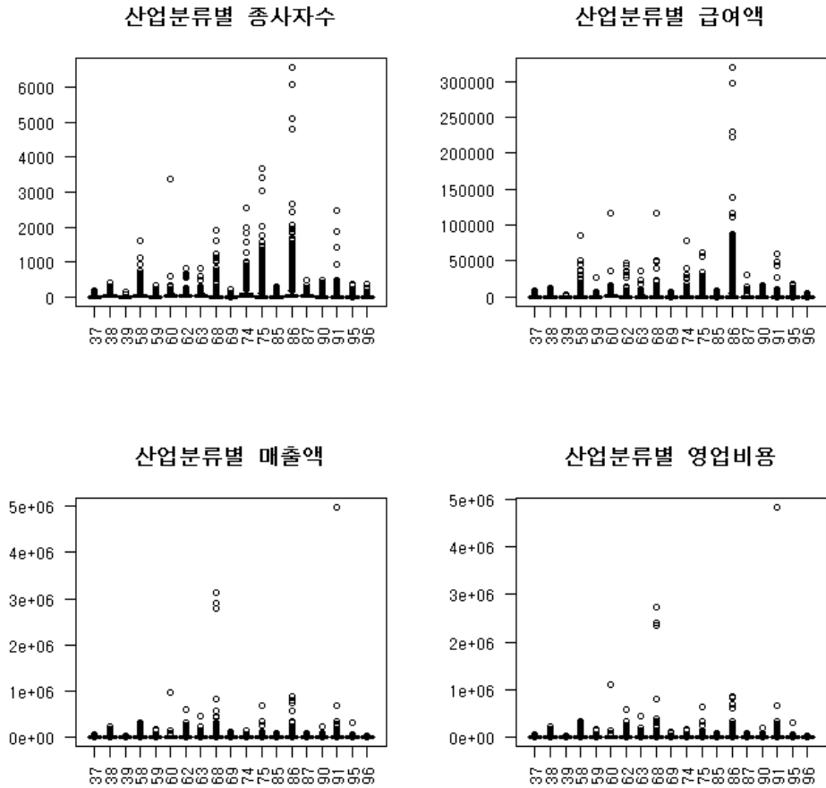
[그림 2-2] 산업분류별 주요항목의 상자그림
