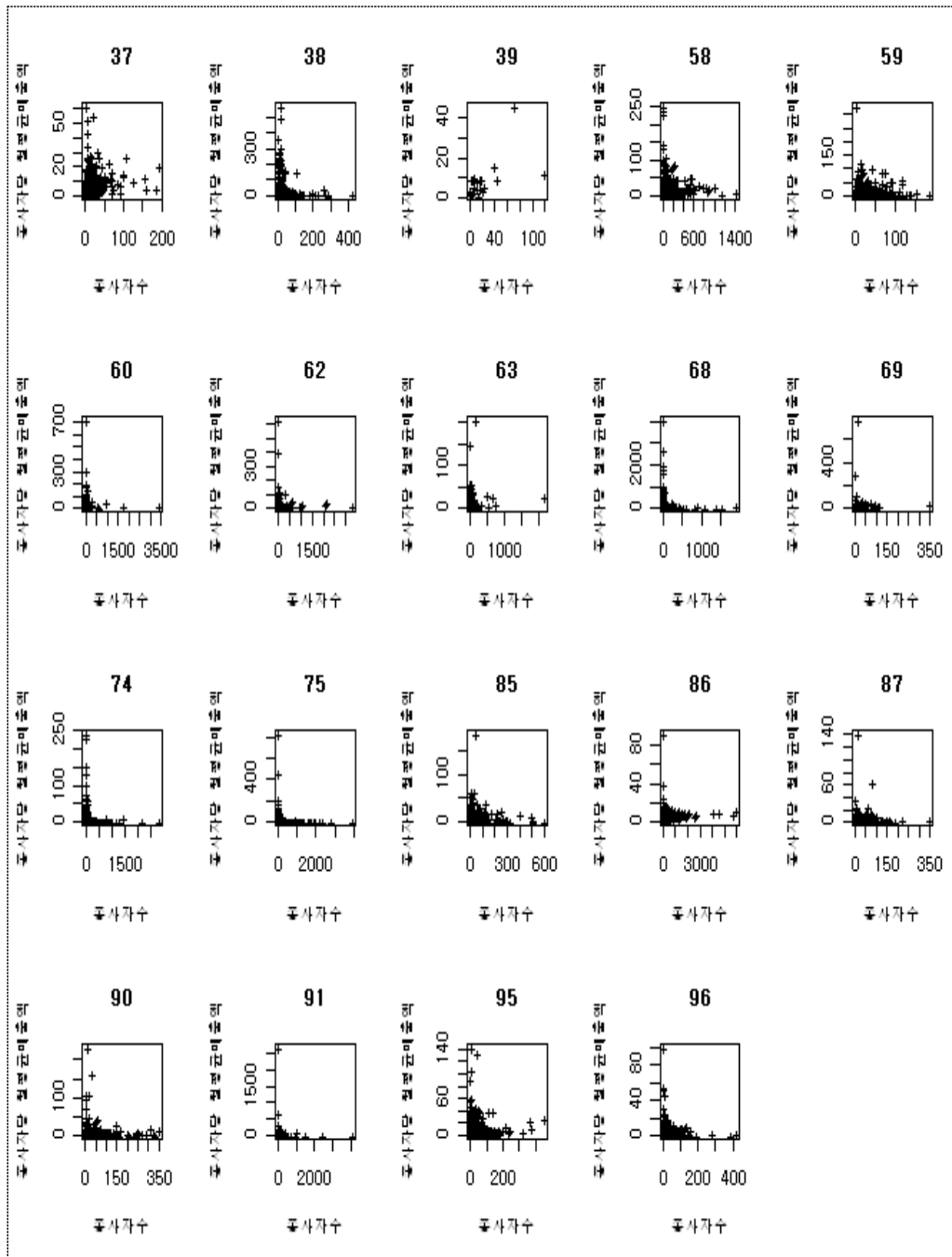
[그림 2-7] 2007년 기준 산업분류별 종사자 1인당 월평균 매출액
