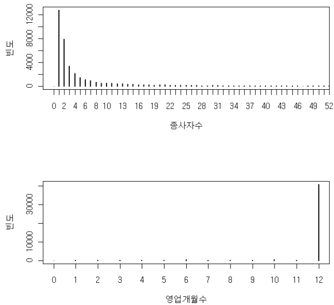
[그림 2-1] 종사자수와 영업개월수의 분포
