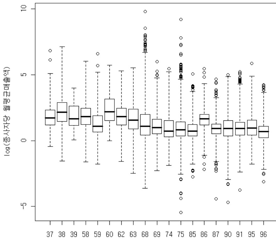
로그변환된 종사자당 월평균매출액의 산업분류별 상자그림 ( 3 \times IQR 사용)
