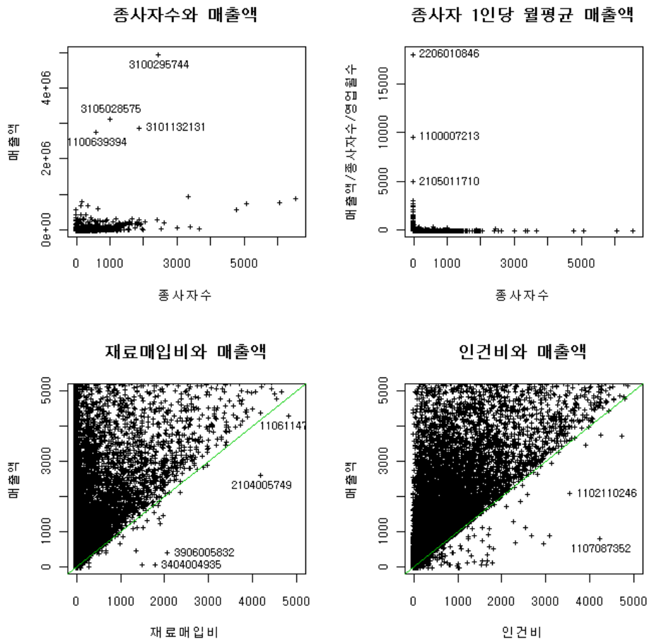
[그림 2-3] 매출액 관련 산점도
