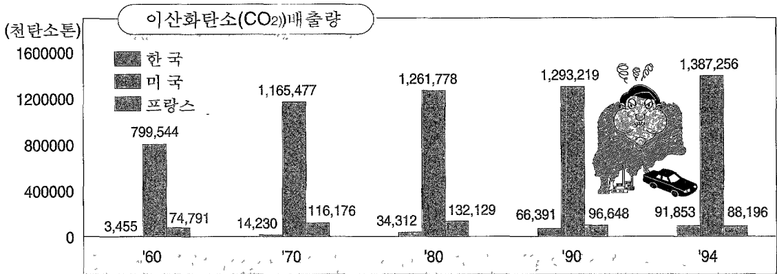
이산화탄소(CO 2 ) 배출량
