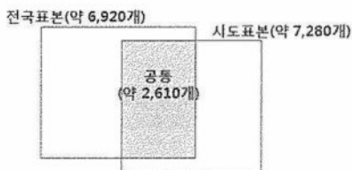
[그림 5] 전국표본과 시도표본 구조
