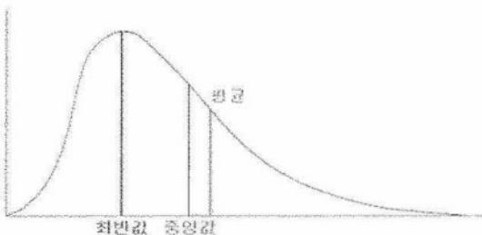
[그림 9] 양(+)의 비대칭분포(Positively skewed)
