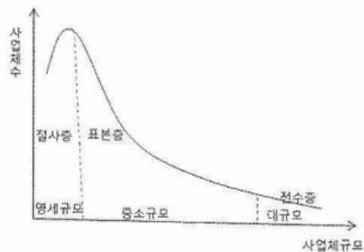
[그림 2] 사업체 모집단의 비대칭분포를 이용한 표본설계방법
