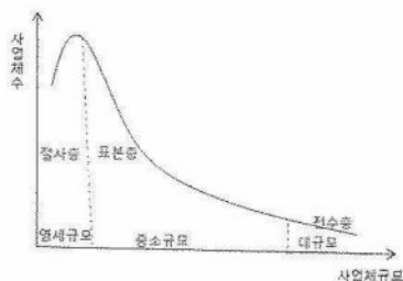
[그림 10] 사업체 모집단의 비대칭분포를 이용한 표본설계방법
