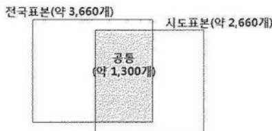
[그림 13] 전국표본과 시도표본 구조
