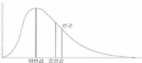
<그림 1> 양(+)의 비대칭분포(Positively skewed)
